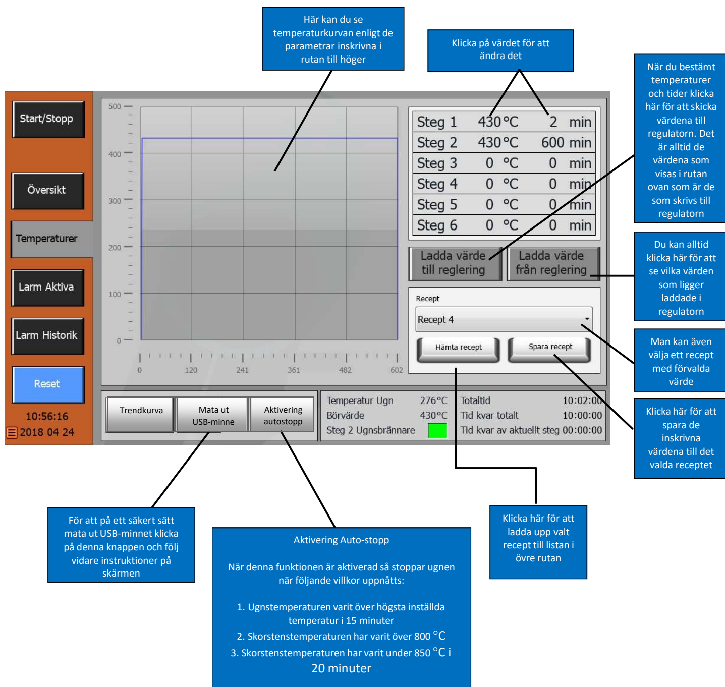
Figur 2 – Säkerhetssystemets utseende vid uppstart av pyrolysuugn
